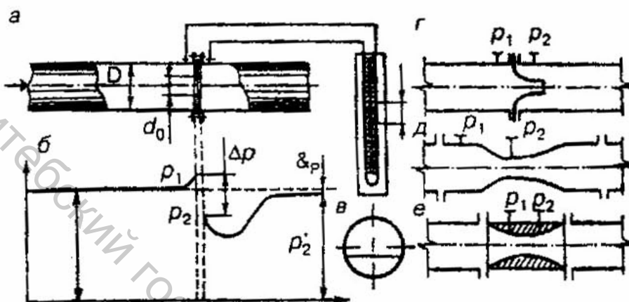
Рис. 7.11. Дроссельные датчики: а- схема, б- определение скорости и расхода, в- сегментная диафрагма, г- сопло, д, е – трубы Вентури и Фостера
