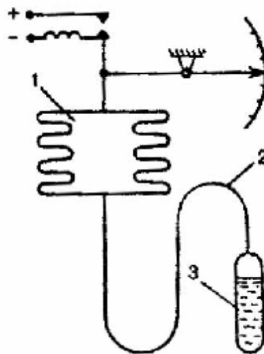
Рис. 7.5. Схема манометрического термометра
