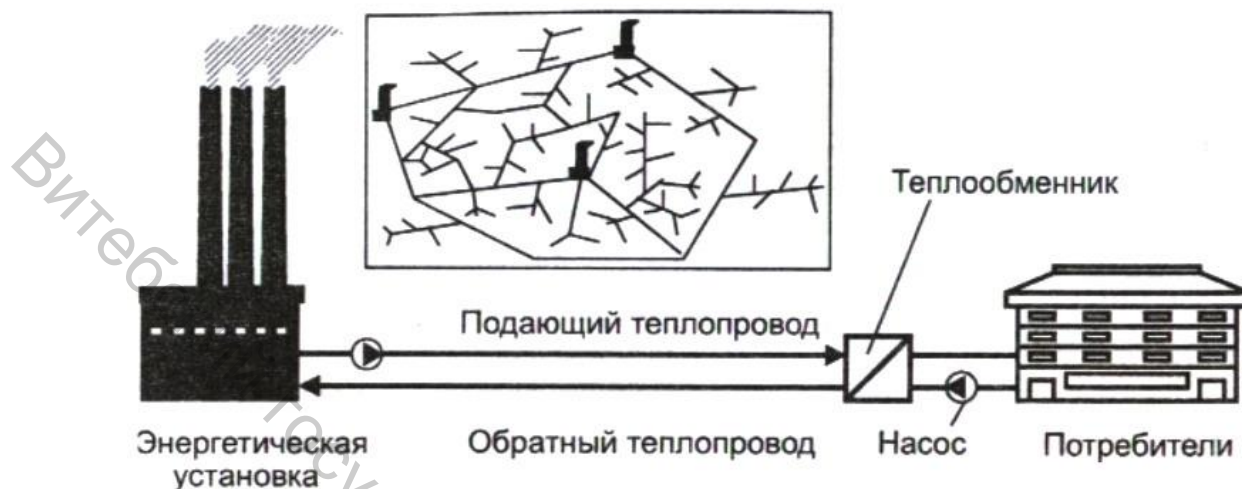
Рис. 4.1. Принципиальная схема централизованного теплоснабжения и тепловой сети
