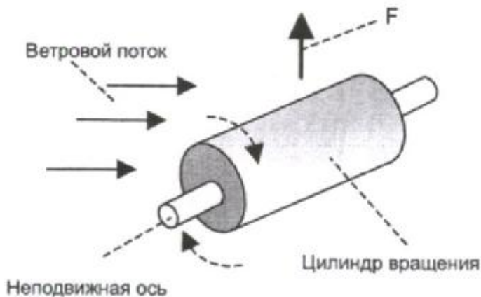
Рис. 3.8. Роторный элемент ветровой установки, использующий эффект Магнуса: F - реактивная подъемная сила
