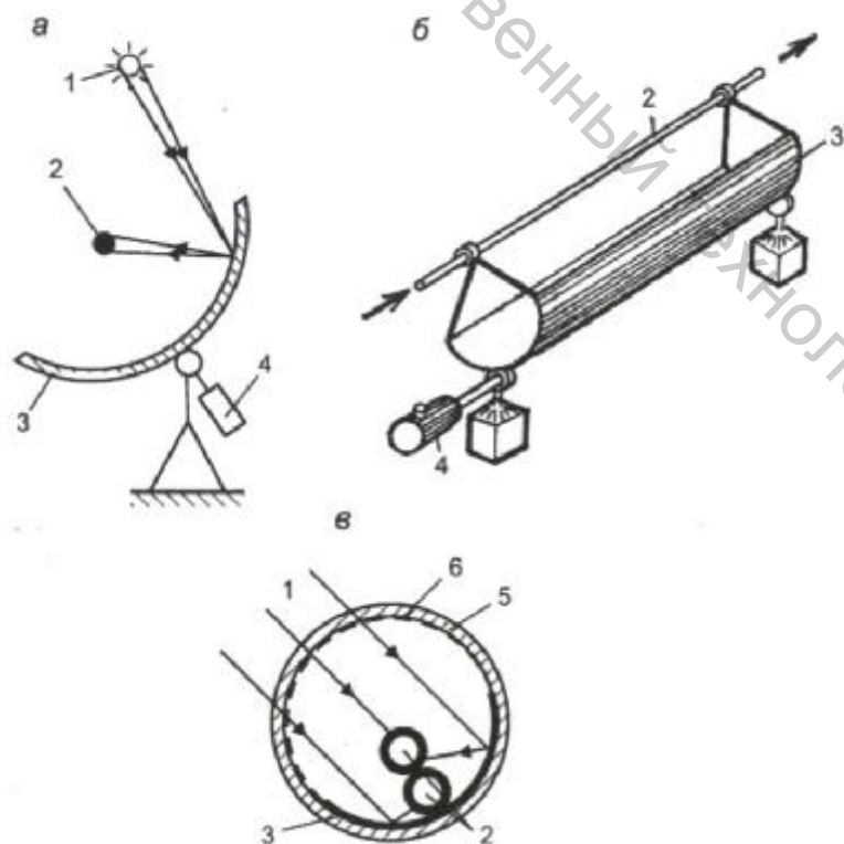
Рис. 3.15. Схемы солнечных коллекторов с концентраторами. Сечение параболического концентратора (а) и его общий вид (б), концентратор с вакуумной трубой (в): 1 - солнце (солнечные лучи); 2 - теплоприемник; 3 - концентратор; 4 - следящее устройство; 5 - вакуумная труба; 6 - селективное покрытие
