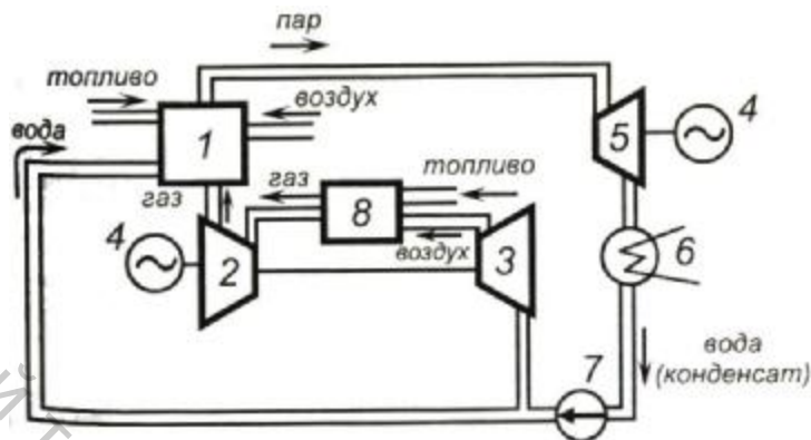
Рис. 2.5. Схема ТЭС с парогазовой установкой с выбросом отработанных газов в паровой котел.
