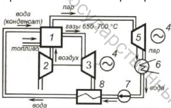
Рис. 2.4 Принципиальная схема ТЭС с парогазовой установкой,
