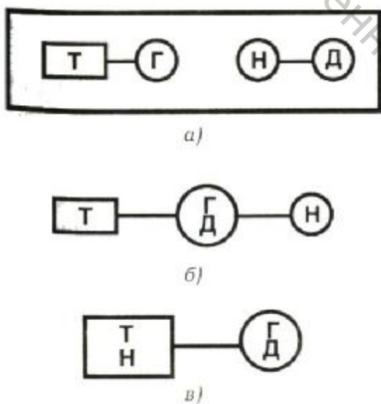
Рис. 2.8. Компоновки ГАЭС.
