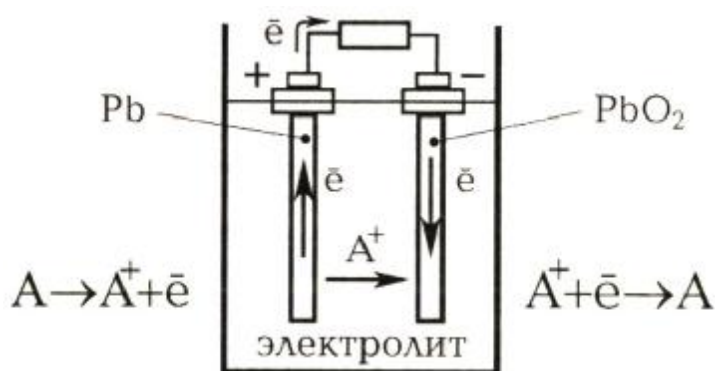
Рис. 2.11. Принципиальная схема электрохимического элемента.
