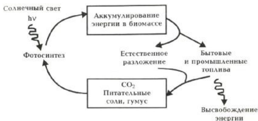
Рис. 3.2. Система планетарного круговорота биомассы
