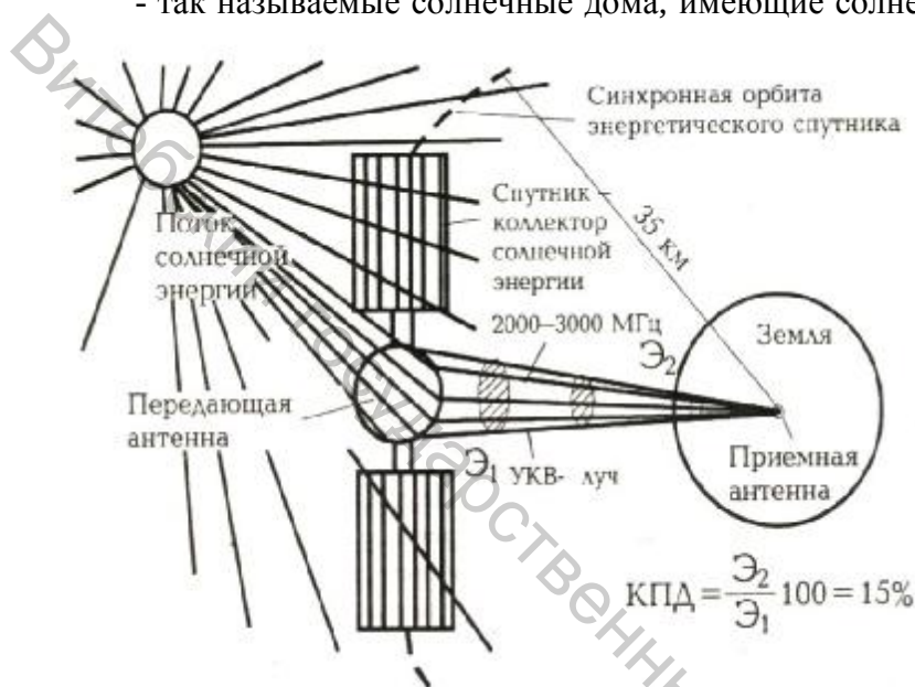
Рис. 3.18. Схема солнечной электростанции на искусственно» спутнике.
