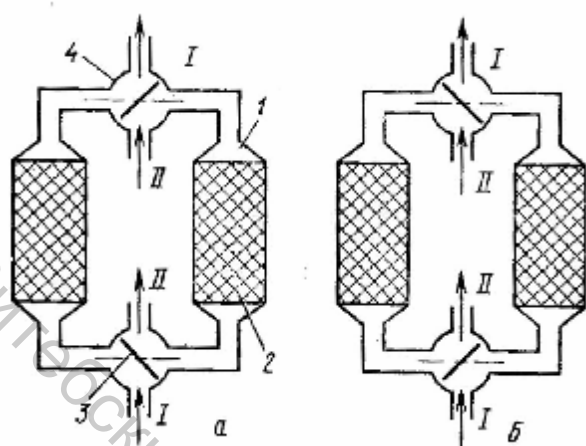
Рис. 8.7. Схемы регенеративных теплообменников: а- левый корпус –период нагрева, б- правый- период охлаждения. 1- корпуса, 2- насадки, 3- перекидные клапана, 4- клапанные коробки
