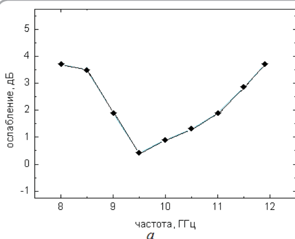
Рисунок 2 – Экранирующие характеристики ткани с покрытием из Cu:
