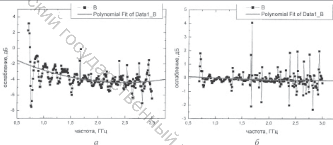
Рисунок 5 – Значения коэффициентов ослабления ЭМИ в диапазоне 0,7–3 ГГц: а – покрытия, осажденные в вакууме; б – покрытия, осажденные в среде CO_2
