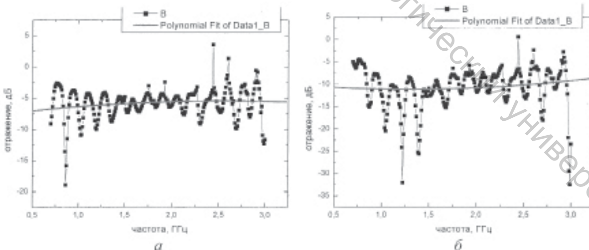
Рисунок 6 – Значения коэффициентов отражения в диапазоне 0,7–3 ГГц: а – покрытия, осажденные в вакууме; б – покрытия, осажденные в среде CO_2
