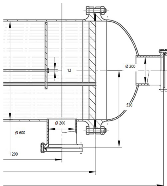
Рисунок 6 – Графическая часть проектируемого теплообменного аппарата
