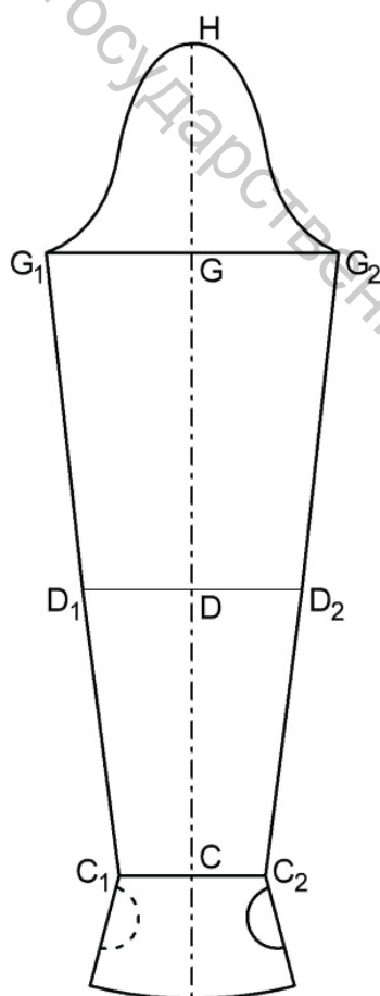
Рисунок 5 – Конструкция детали компрессионного рукава, нижняя часть которого выполнена по варианту 2
