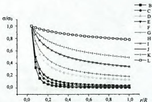
Рис. 2. Распределение прочности для бумаги различных видов: В — бумага АО «Волга»; С — Балахнинского ЦБК; D — цветная бумага Балахнинского ЦБК; E — офсетная бумага №1; F — Люми Силк; G — Юнион Арт; H — Юнион Силк; I — Дата Копи; J — картон Малмеро; K — бумага Кондопогского ЦБК; L — Люми Арт.
