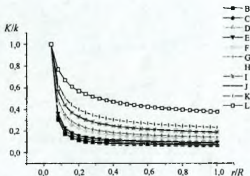
Рис. 1. Распределение объемных модулей упругости для бумаги различных видов: В — бумага АО «Волга»; С — Балахнинского ЦБК; D — цветная бумага Балахнинского ЦБК; E — офсетная бумага №1; F — Люми Силк; G — Юнион Арт; H — Юнион Силк; I — Дата Копи; J — картон Малмер; K — бумага Кондопогского ЦБК; L — Люми Арт.
