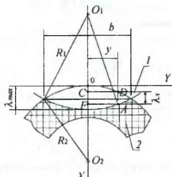
Рис. 3. Схема деформации упругой покрышки цилиндра: 1 — жесткий цилиндр, 2 — цилиндр с эластичной оболочкой; R_{1,2} — радиусы жесткого и цилиндра с эластичной оболочкой.
