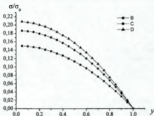
Рис. 5. Зависимость напряжения от деформации для однослойного декельного материала из неплавленого вулканизата (30 вес. частей сажи): B — E = 2,30 МПа; C — E = 2,85 МПа; D — E = 3,18 МПа.
