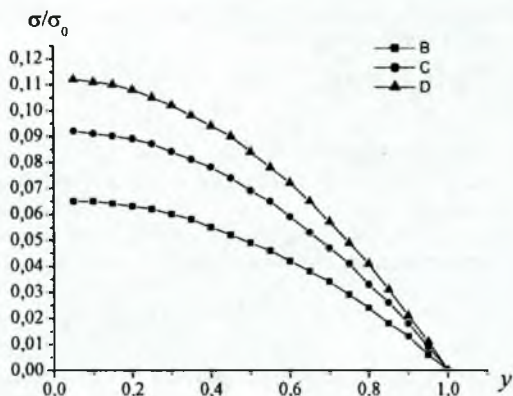
Рис. 4. Зависимость напряжения от деформации для однослойного декельного материала из неплавленого вулканизата: B — E = 1,00 МПа; C — E = 1,41 МПа; D — E = 1,71 МПа.
