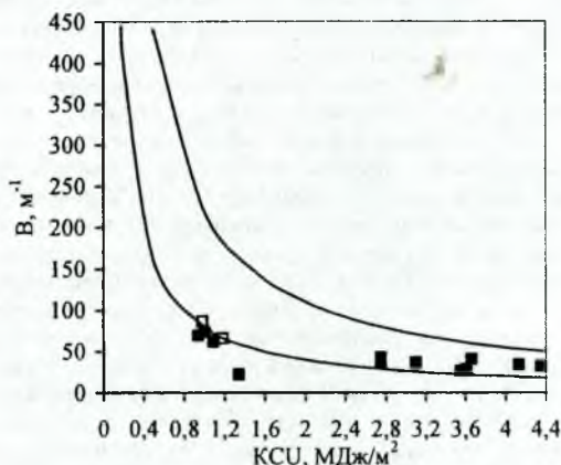
Рис. 4. Результаты оценки деградации механических свойств стали 15Х5М. Условные обозначения: ■ — 15Х5М (после длительной эксплуатации); □ — 15Х5М (минимальные свойства по ГОСТ 550)
