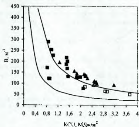
Рис. 3. Результаты оценки дегградации механических свойств аустенитных нержавеющих сталей 08X18H10T и 12X18H10T. Условные обозначения: ■ — 12X18H10T (после длительной эксплуатации); ▲ — 08X18H10T (после длительной эксплуатации); □ — 12X18H10T (по ГОСТ 7350); △ — 08X18H10T (свойства по [6, с. 527])
