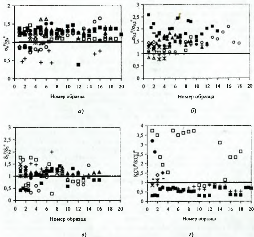
Рис. 1. Результаты оценки годности исследованных материалов по отношению: а) пределов прочности \sigma_B^P/\sigma_B^C (а); пределов текучести \sigma_{0.2}^P/\sigma_{0.2}^C (б); относительных удлинений \delta_5^P/\delta_5^C (в); ударной вязкости KCU^P/KCU^C (г). Условные обозначения: ■ — 12Х18Н10Т; ▲ — 08Х18Н10Т; — — 10Х17Н13М2Г; ◆ — 37Х12Н8Г8МФБ; □ — 15Х5М; ○ — Сталь 20; + — 08Х13; . — 30Х13; ◇ — 09Г2С; — — 14Г2; × — Ст3сп; • — Ст3.
