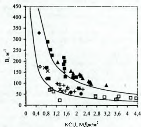
Рис. 2. Результаты оценки дегградации механических свойств анализируемого металла при помощи метода графической интерпретации характеристик механических свойств стали. Условные обозначения: см. пояснения к рис. 1
