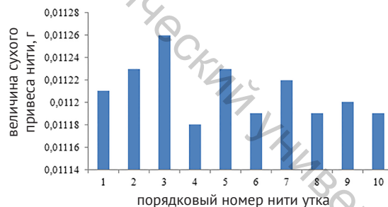
Рисунок 4 – Величина сухого привеса различных нитей утка тканой основы композиционного материала при концентрации стирол-акрилата – 500 г/л
