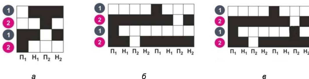
Рисунок 3 – Модельные переплетения для изготовления изделий на ткацком станке.
